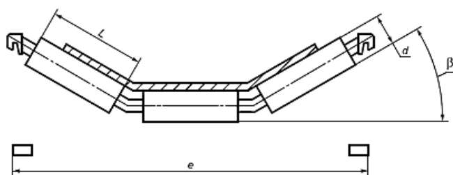
Рисунок 1 - Жесткая трехроликовая опора
