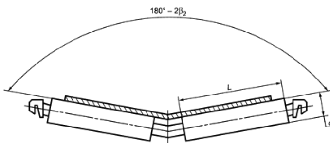
Рисунок 3 - Жесткая двухроликовая опора
