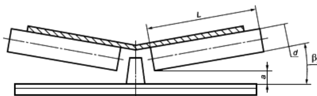
Рисунок 2 - Трехроликовая гирляндная опора
