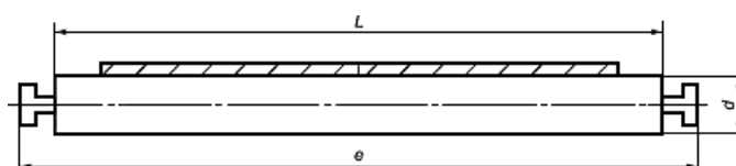
Рисунок 4 - Двухроликовая гирляндная опора
